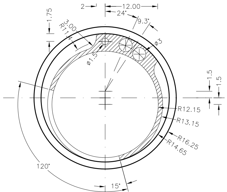
Seccion
