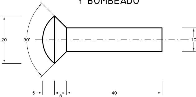
REMACHE DE CABEZA AVELLANADA Y BOMBEADO
