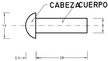
REMACHE DE CABEZA REDONDA
