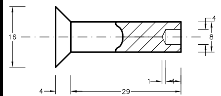
REMACHE DE CABEZA AVELLANADA A 90° Y CUERPO PERFORADO
