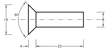
REMACHE DE CABEZA AVELLANADA A 90°
