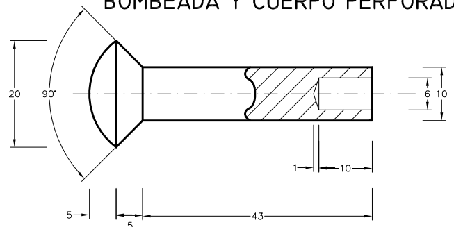
REMACHE DE CABEZA AVELLANADA BOMBEADA Y CUERPO PERFORADO
