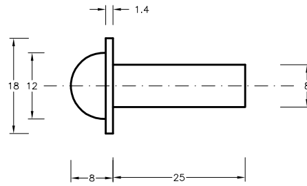
REMACHE DE CABEZA REDONDA CON REBABA Y REDONDEAMIENTO
