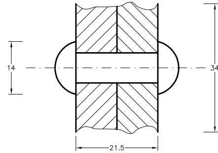
PIEZAS REMACHADAS
